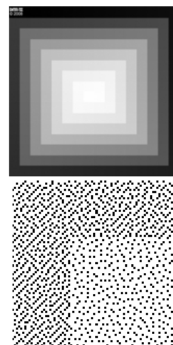
Abb. 1: Oben das RWBK 1.0 in Originalgröße (bei 2540 dpi Bebilderungsauflösung), unten ein stark vergrößerter Ausschnitt daraus, der die mikroskopischen Strukturen deutlich zeigt
